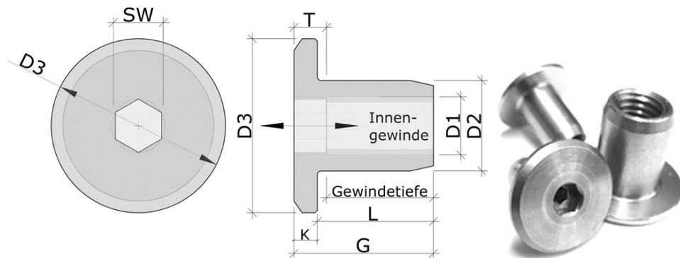
Hülsmutter Flachkopf 3228 © kury.de
